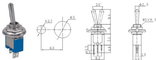
BTS-102 ON-ON SPDT 3P
