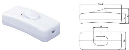
A-TOP5-303-1 SPST A-TOP5-303-2 DPST
