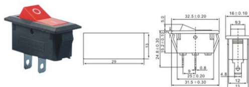
A-TOP3-8-101 ON-OFF A-TOP3-8-102 ON-ON
