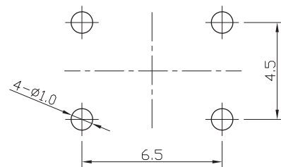
P.C.B LAND DIMENSION
