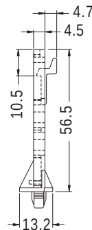
PCB DIM.
