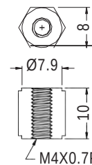
M4X0.7P
