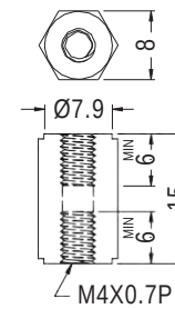
M4X0.7P
