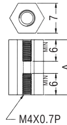
M4X0.7P
